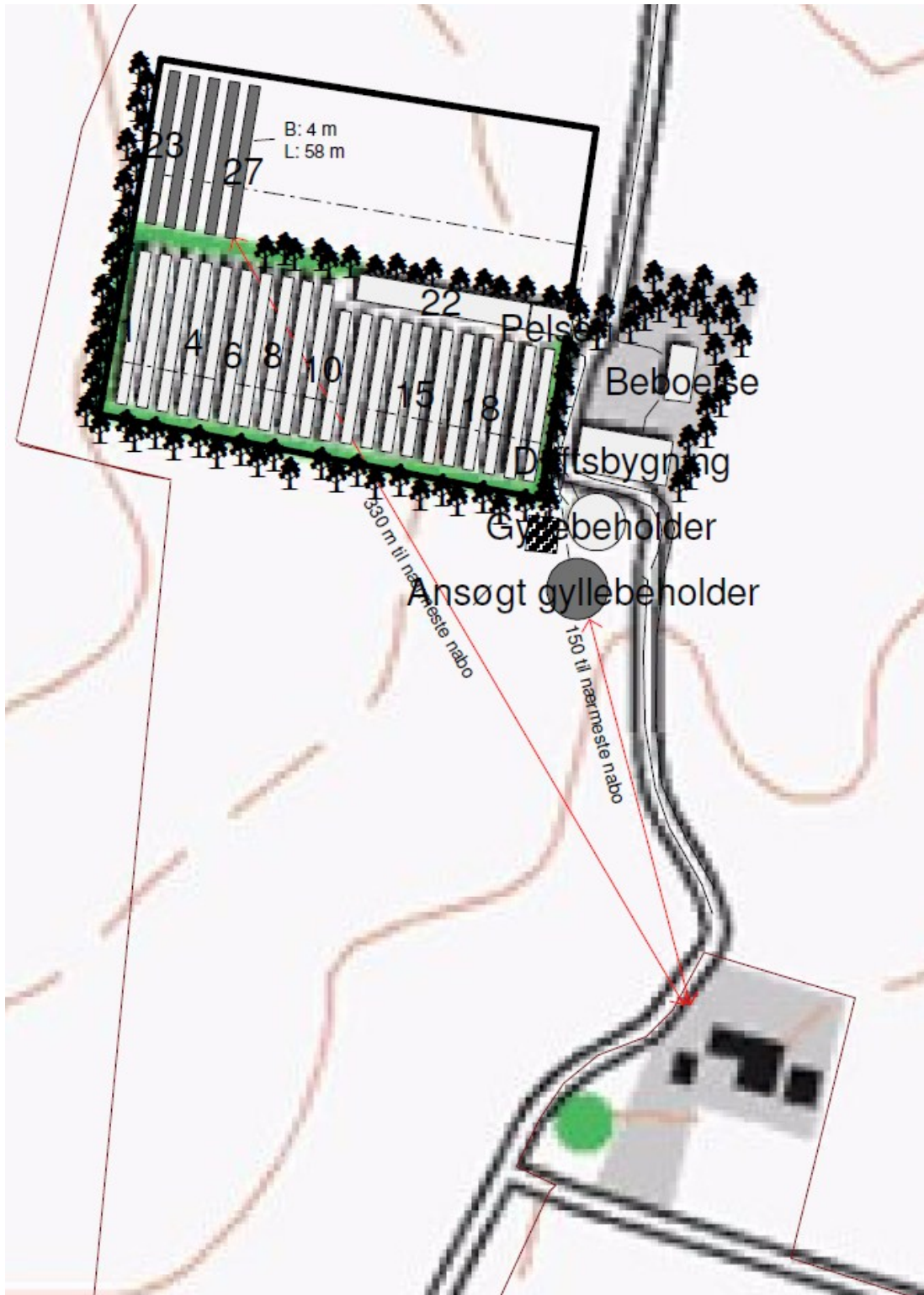
Figur 1. Placering af gyllebeholder samt rørføringen til denne på Grætrupvej 2.
